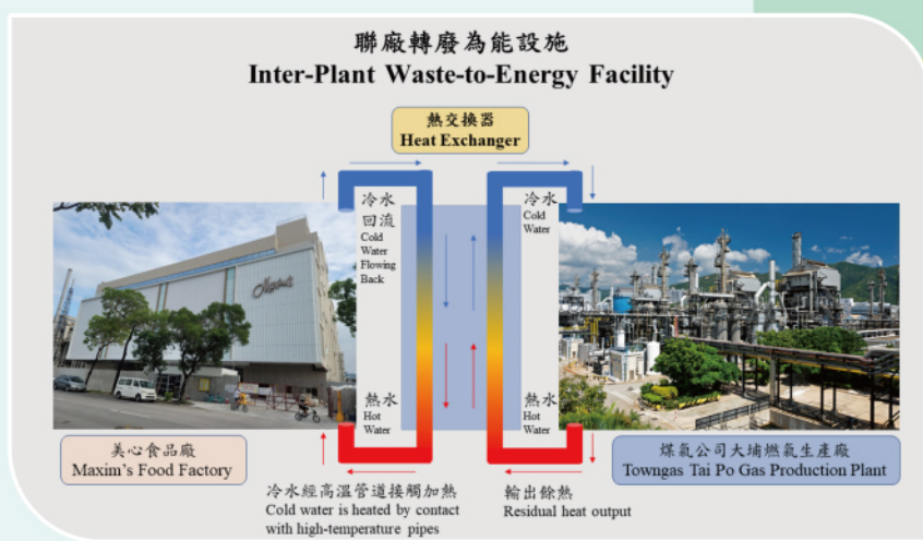
▲ 透過兩廠之間的熱交換器，煤氣公司把收集得到的製氣餘熱，輸送到美心食品廠。
